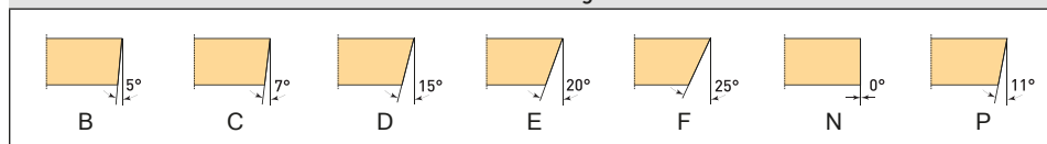
2 - Relief angle
