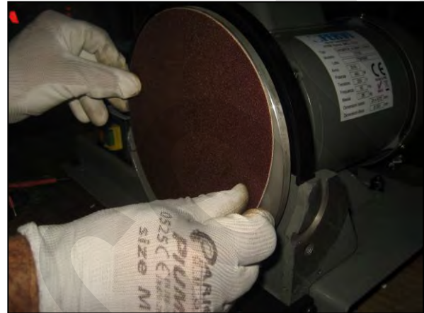
Figura 12 – Montaggio disco
